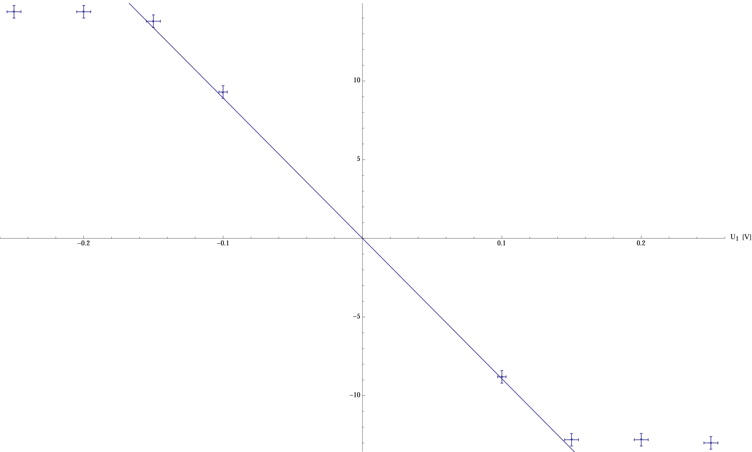
Aufgabe 1 (a): R_G = 274 \text{ k}\Omega U_A [V]
