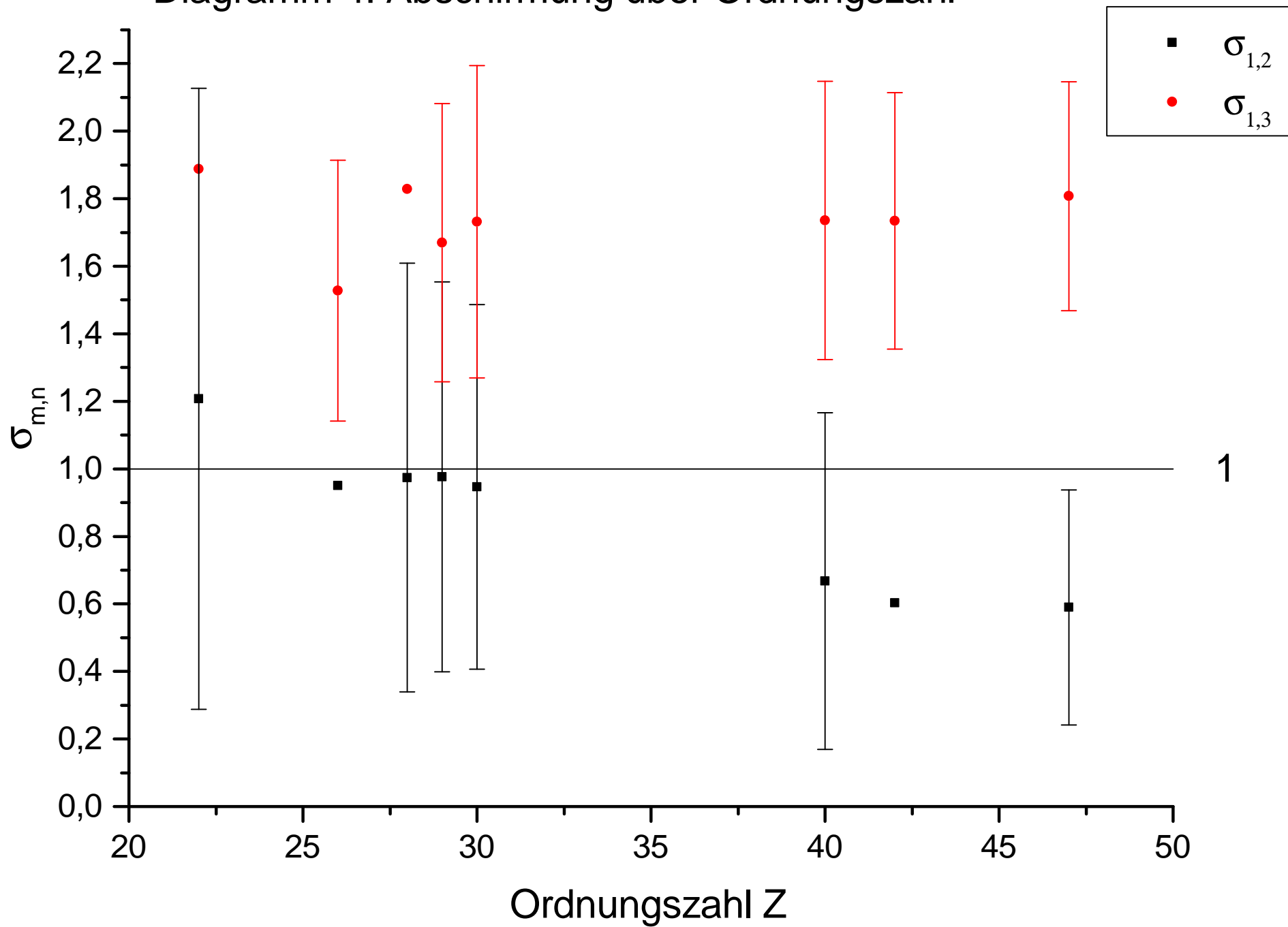
Diagramm 4: Abschirmung über Ordnungszahl
