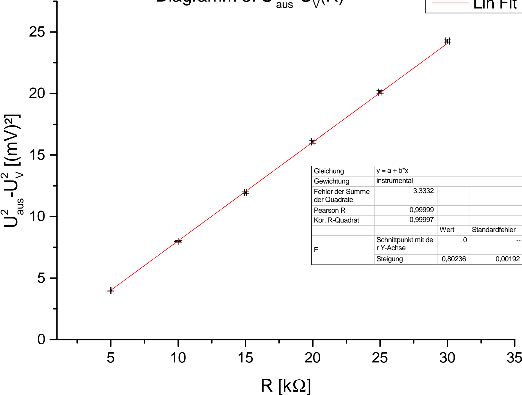
Diagramm 3: U_{\text{aus}}^2 - U_{\text{V}}^2(R)
